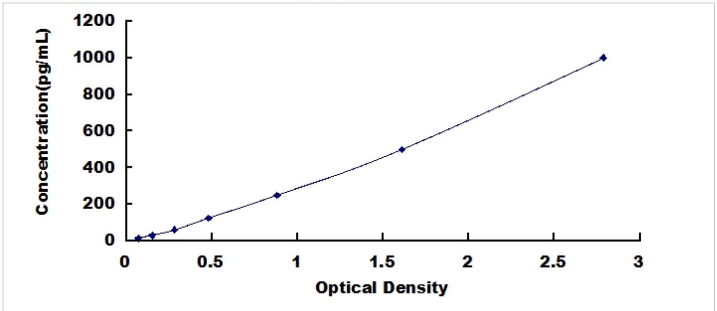
兔白介素 8 (IL8) 检测试剂盒标准曲线
