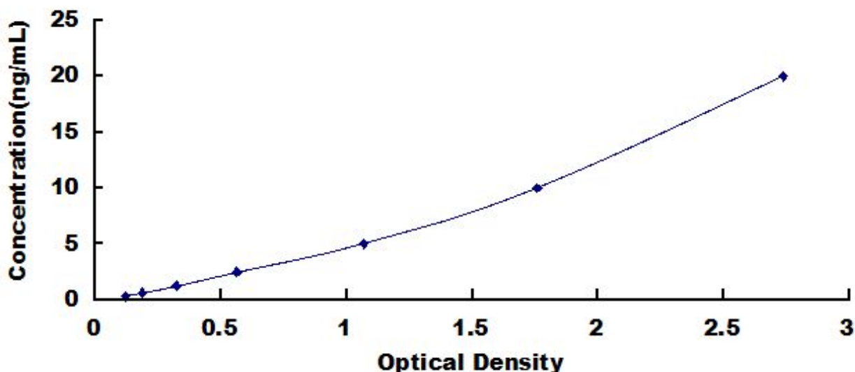
小鼠血管生长素(ANG)检测试剂盒标准曲线
