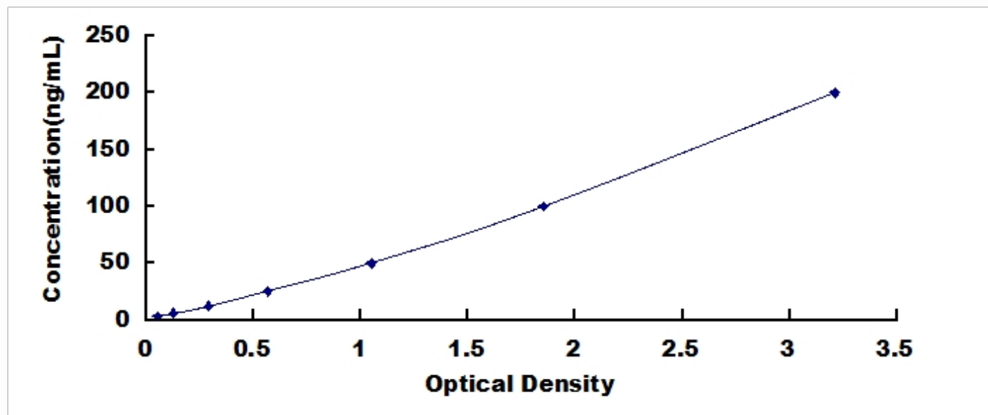
人抗肿瘤坏死因子 \alpha (Anti-TNF \alpha ) 检测试剂盒标准曲线
