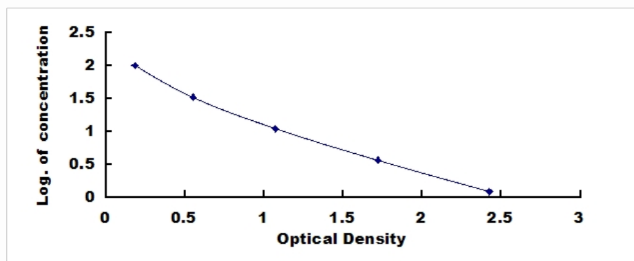
胆红素(Bb)检测试剂盒标准曲线
