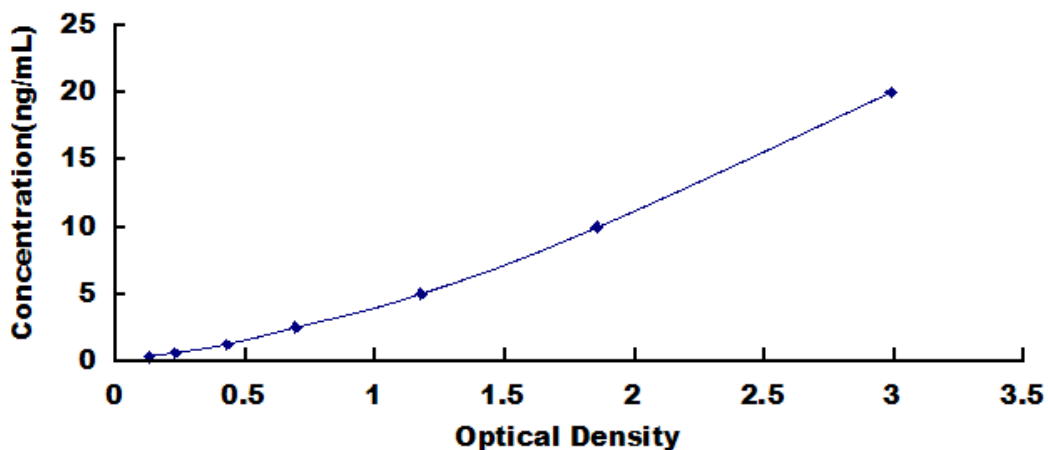
人补体成分 1r (C1r) 试剂盒标准曲线
