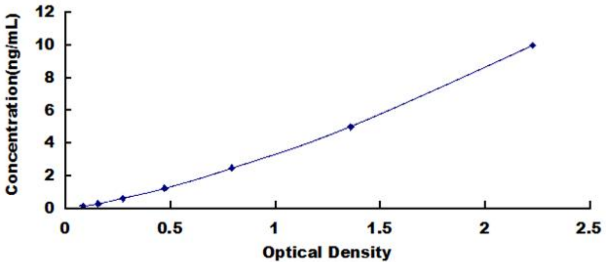
人周期素依赖性激酶抑制因子 1A (CDKN1A) 检测试剂盒标准曲线
