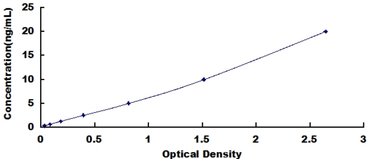
大鼠细胞色素 P450 家族成员 2C9 (CYP2C9) 检测试剂盒标准曲线
