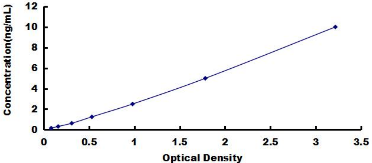
人 Duffy 血型趋化因子受体 (DARC) 检测试剂盒标准曲线
