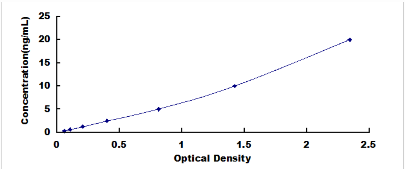
小鼠 G 蛋白偶联受体激酶 5 (GRK5) 检测试剂盒标准曲线
