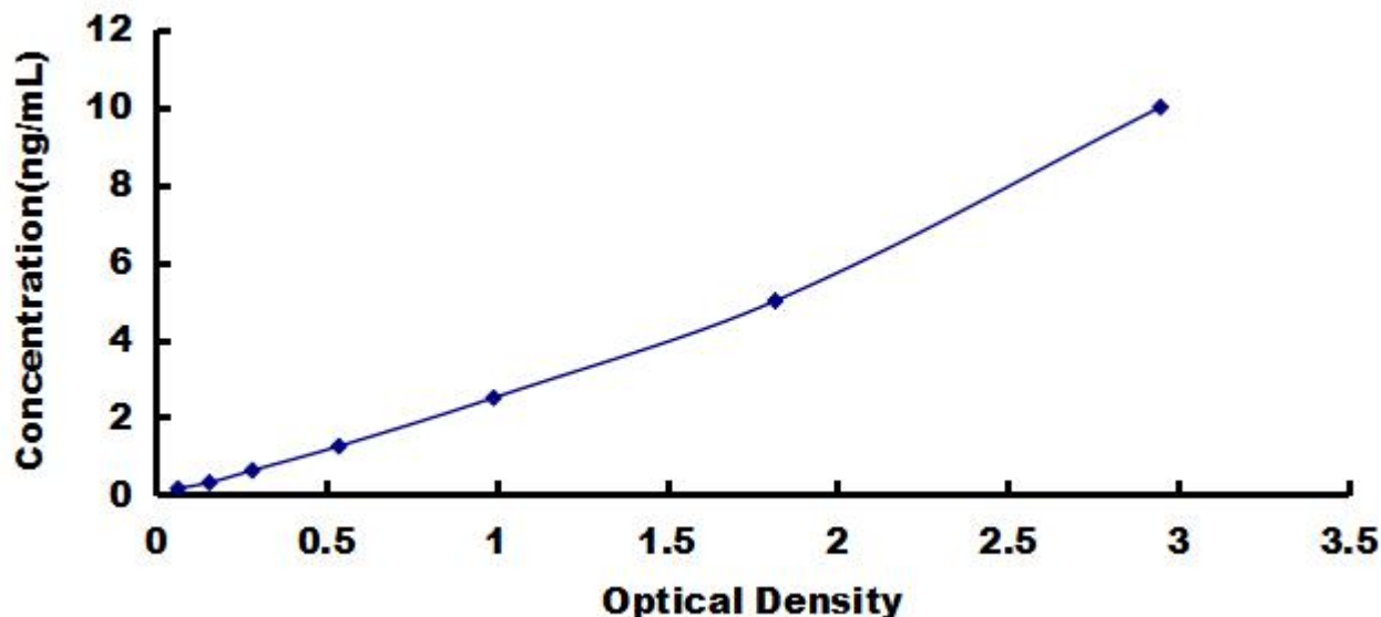
猪半乳糖凝集素 1 (GAL1) 检测试剂盒标准曲线
