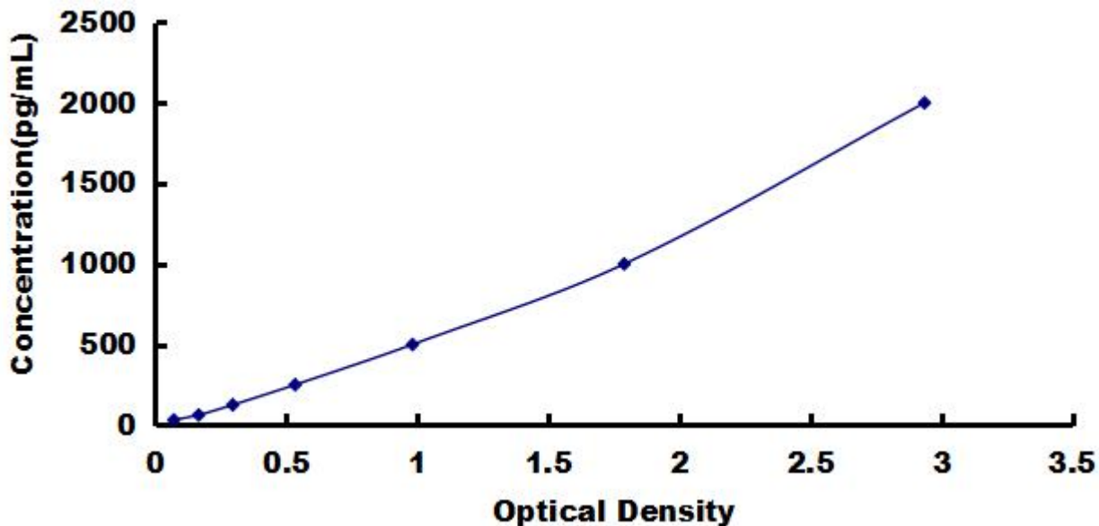
人干扰素诱导跨膜蛋白 3 (IFITM3) 检测试剂盒标准曲线
