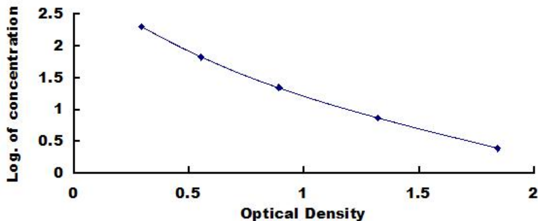
犬尿酸 (KYN) 检测试剂盒标准曲线
