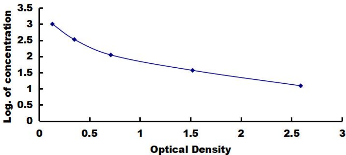
大鼠成骨生长肽 (OGP) 检测试剂盒标准曲线
