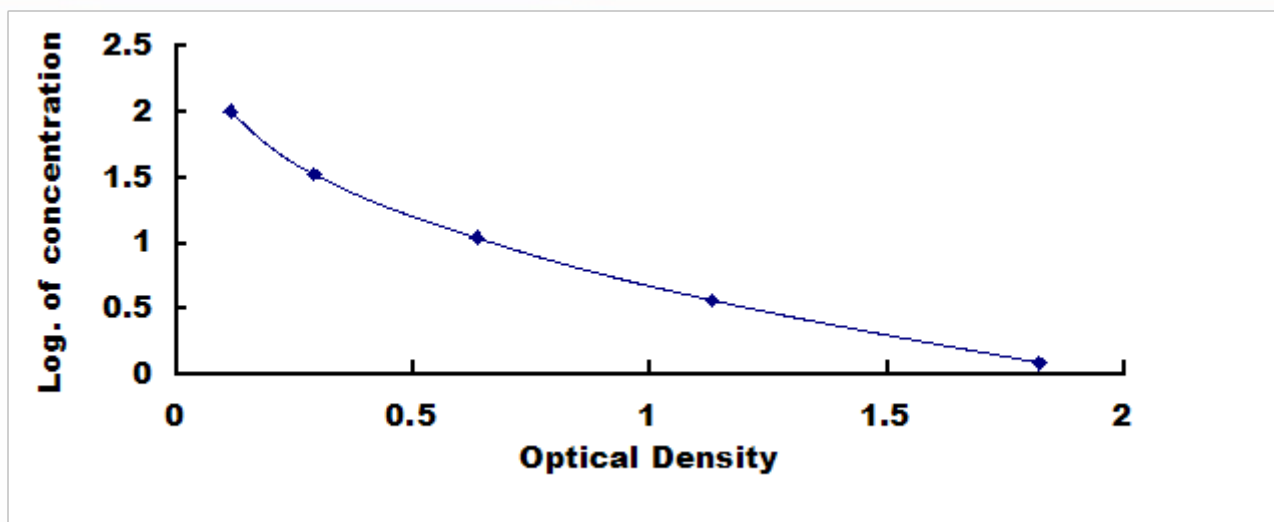
喹啉酸(QA)检测试剂盒标准曲线
