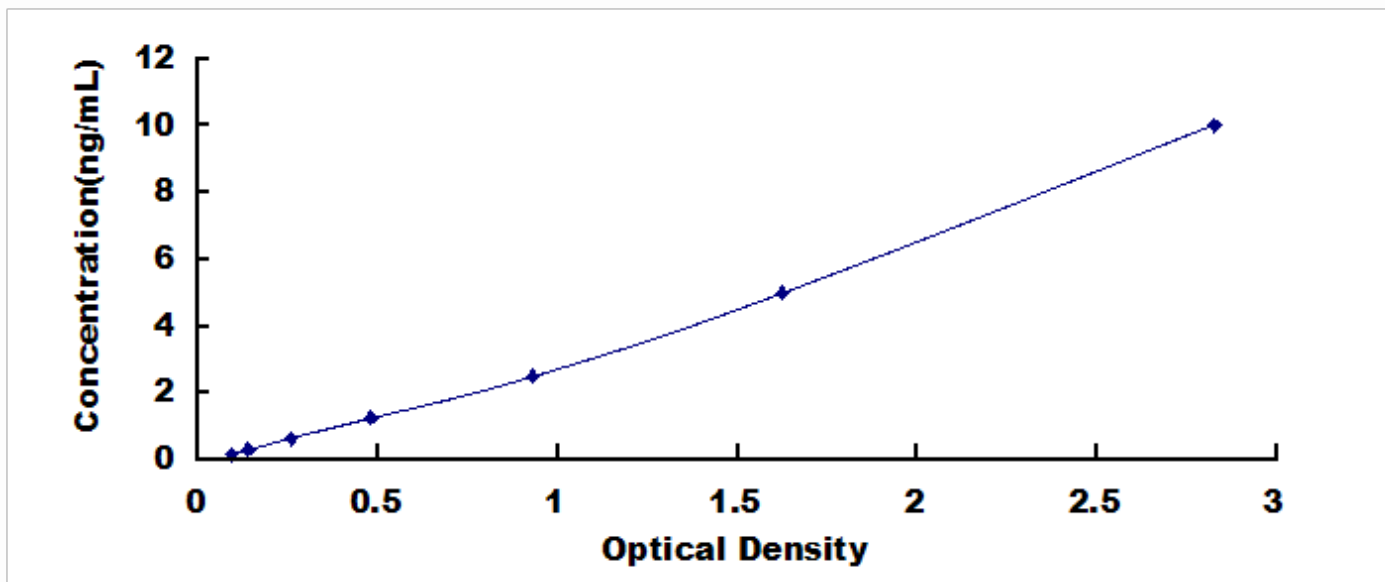
人松弛素/胰岛素样肽受体 3 (RXFP3) 检测试剂盒标准曲线
