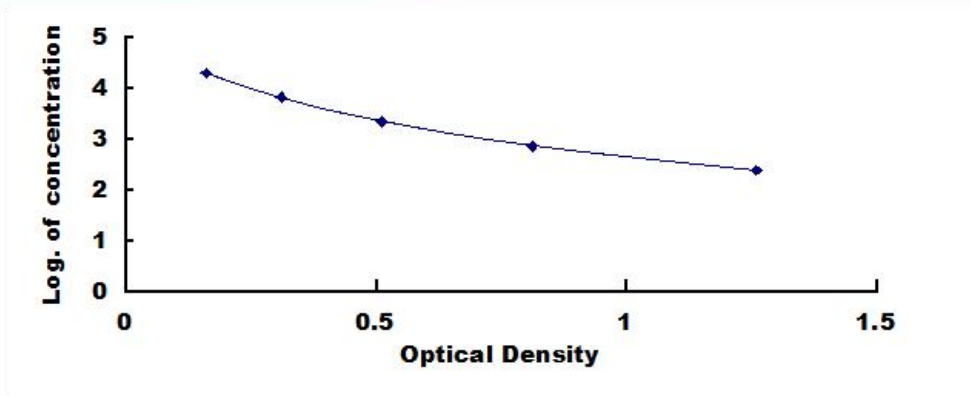
白藜芦醇 (RVT) 检测试剂盒标准曲线
