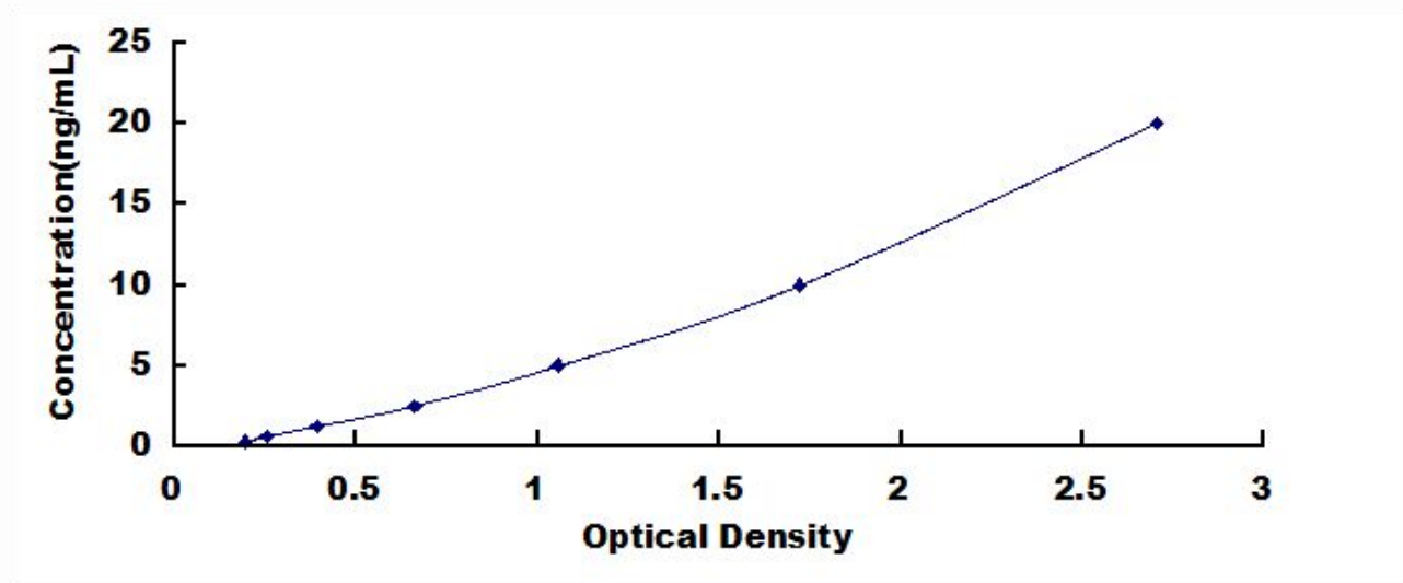
小鼠硫酸酯酶 2 (SULF2) 检测试剂盒标准曲线
