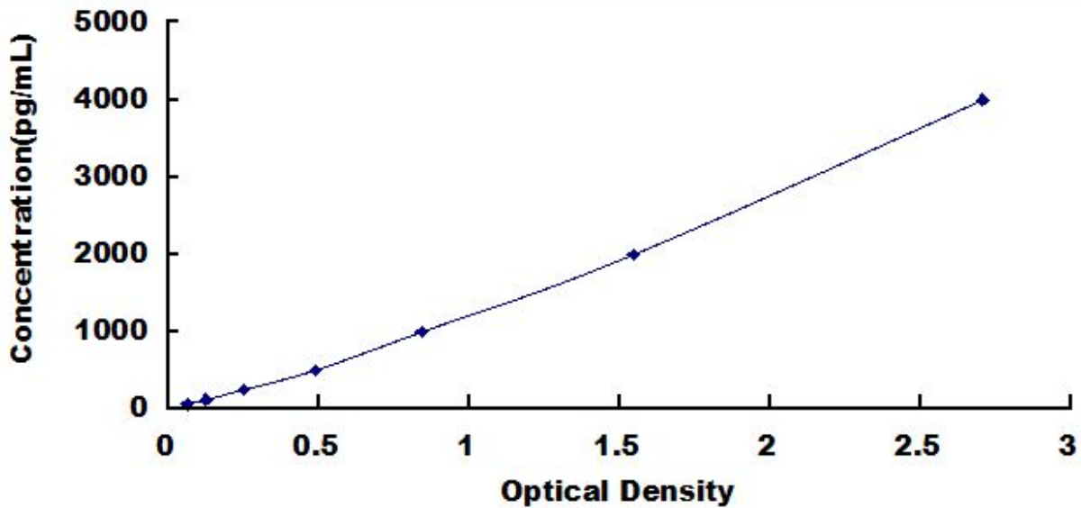
人血管内皮生长因子抑制因子(VEGF)检测试剂盒标准曲线
