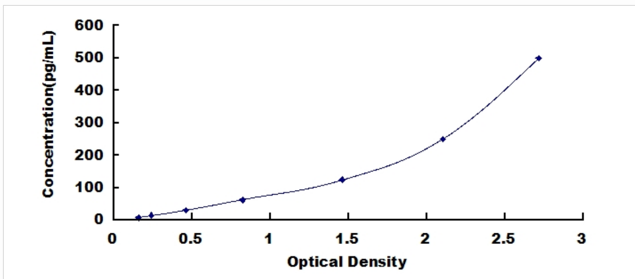
豚鼠肿瘤坏死因子 \alpha (TNF \alpha ) 检测试剂盒标准曲线
