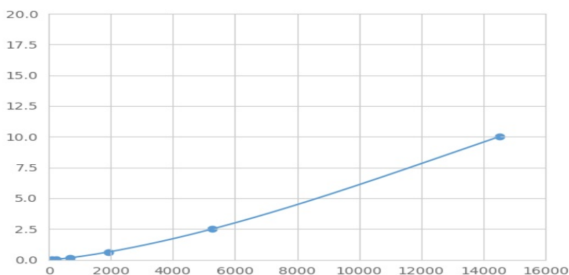
(半胱氨酸蛋白酶抑制剂3)检测试剂盒标准曲线
