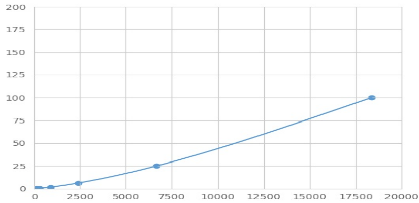
(N-乙酰转移酶1) 检测试剂盒标准曲线
