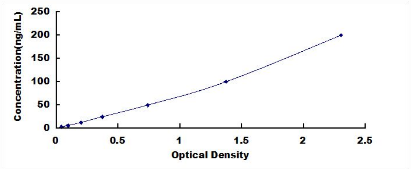
小鼠热休克蛋白 70 (HSP70) 检测试剂盒标准曲线
