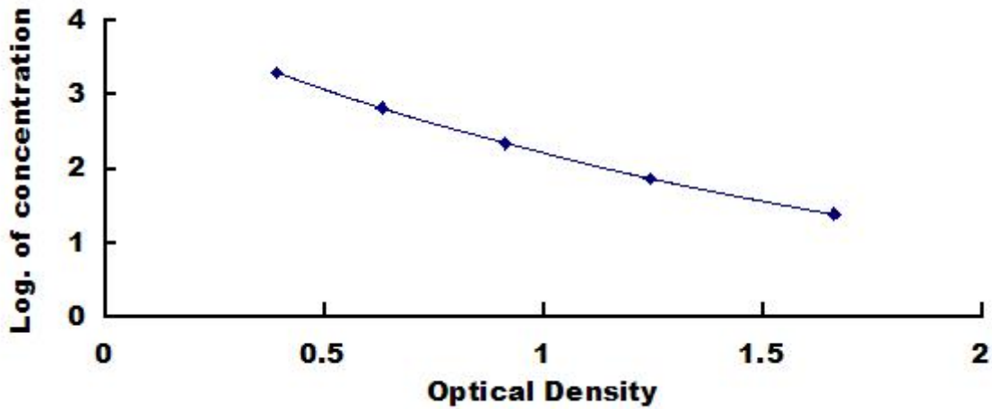
犬尿酸 (KYN A) 检测试剂盒标准曲线
